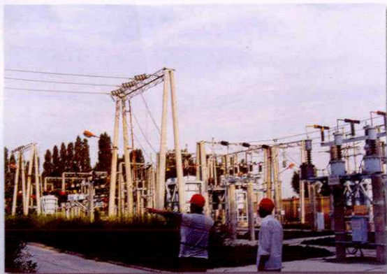
十一万伏变电站（1996 年）
