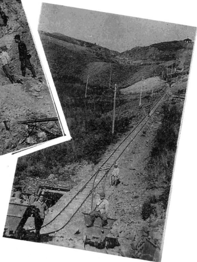
西十五马力卷扬600米坑道
