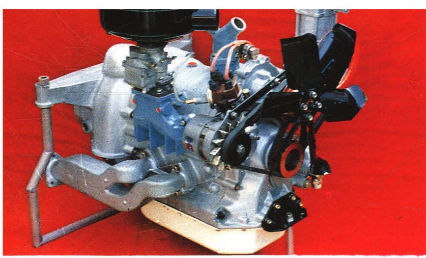
JZ211B型汽车 转子发动机
