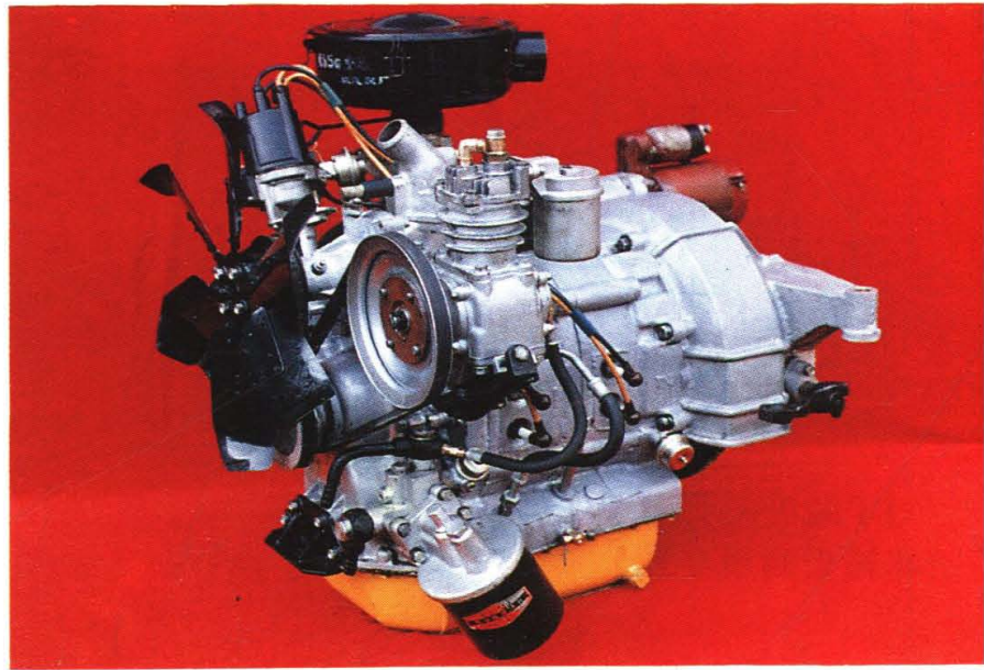
JZ211C型汽车 转子发动机
