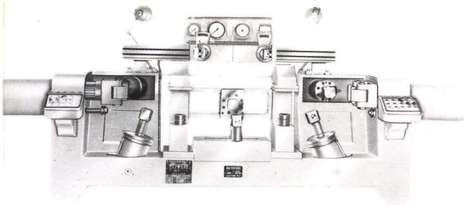
ZJ46-49型汽车 前后桥检验校正机
