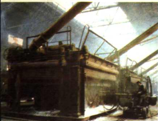
60kA 铝电解系列
