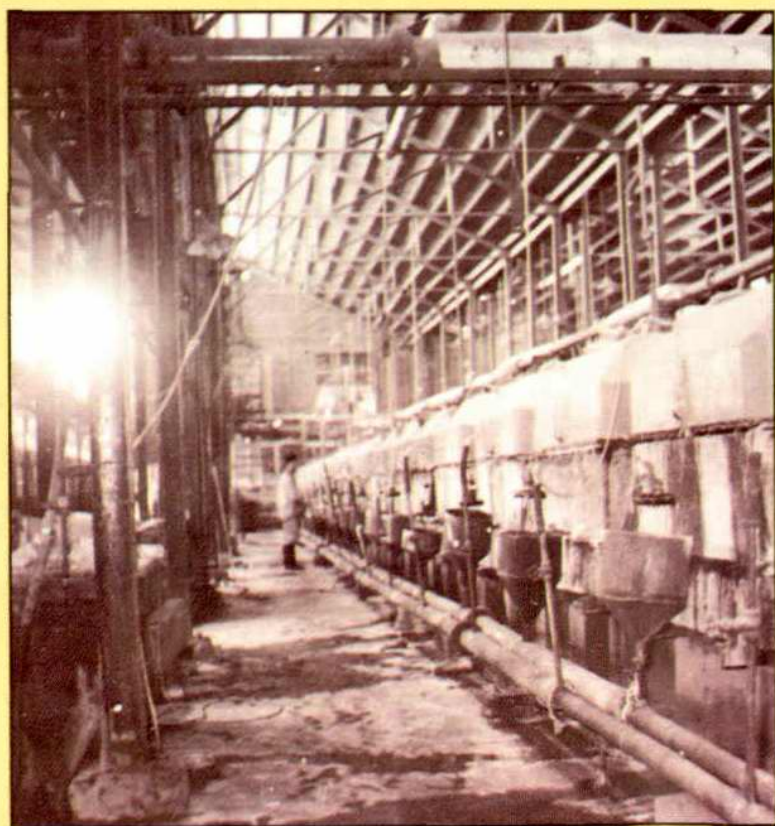
▲ 1960 年立式隔膜电解槽
