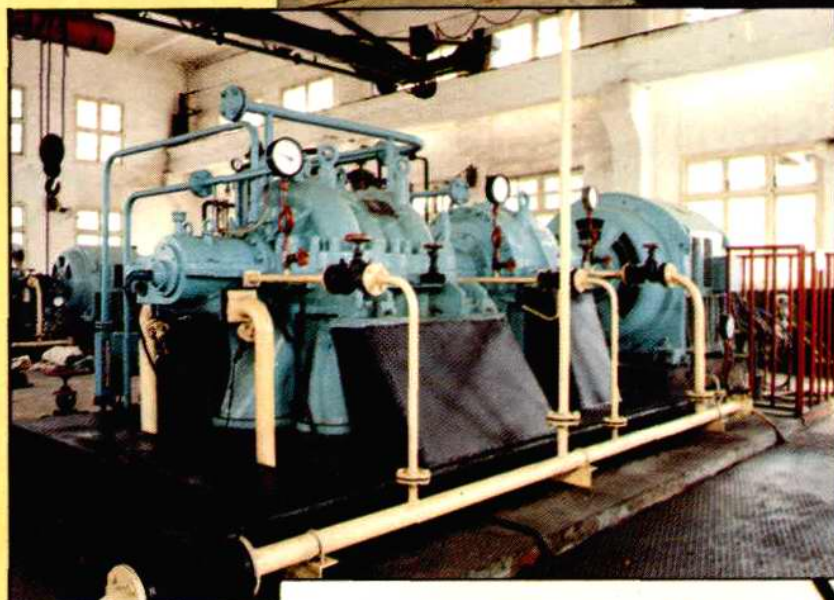
乙稀糊树脂生产装置
