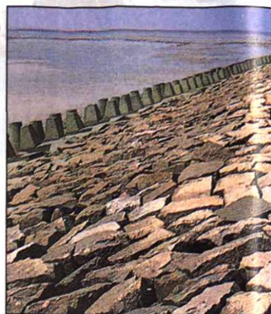
顺坝 Longitudinal dikes
