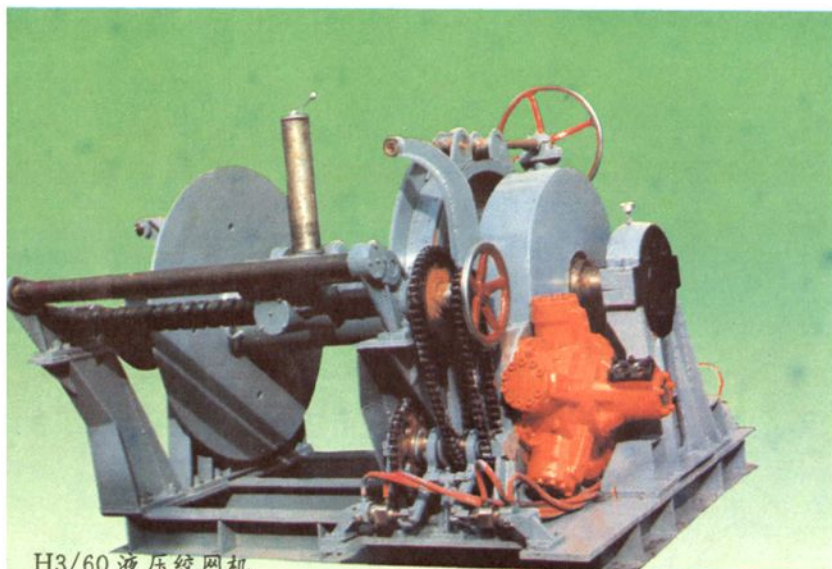
H3/60 液压绞网机
