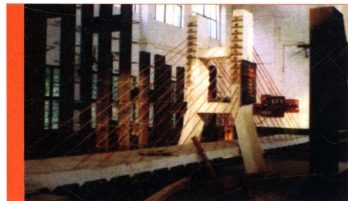
中心实验室能够承担工程材料、工程结构、桩基等试验和检测,图为 1/10 斜拉桥试验
