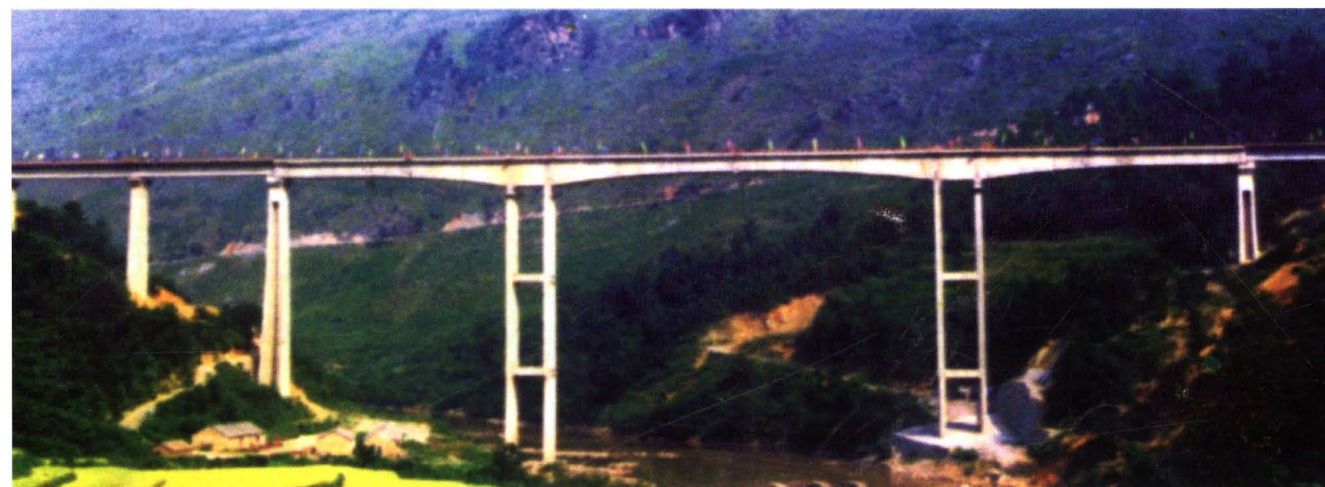
南昆铁路四座新技术桥梁之一——喜旧溪河大桥。我院教师参加设计、科研并负责工程监理及成桥通车鉴定,并因此成为国家科技进步一等奖获奖单位。
