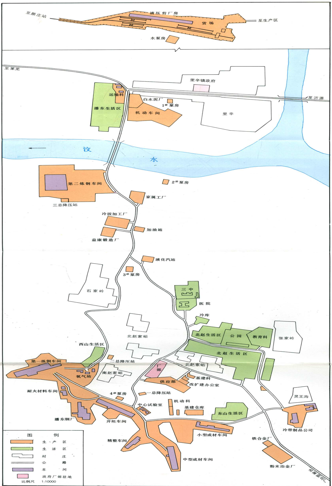
莱钢特殊钢厂平面图
