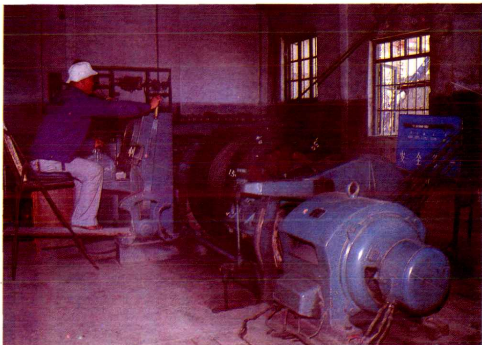
北戴金矿1976年安装的1.2米提升机为招远县地方采金最早的一台
