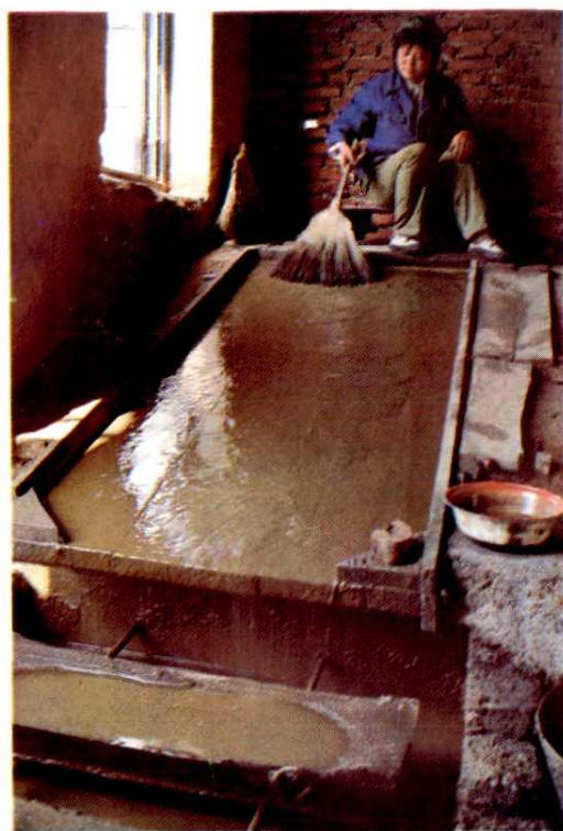
溜槽选矿（拉流）
