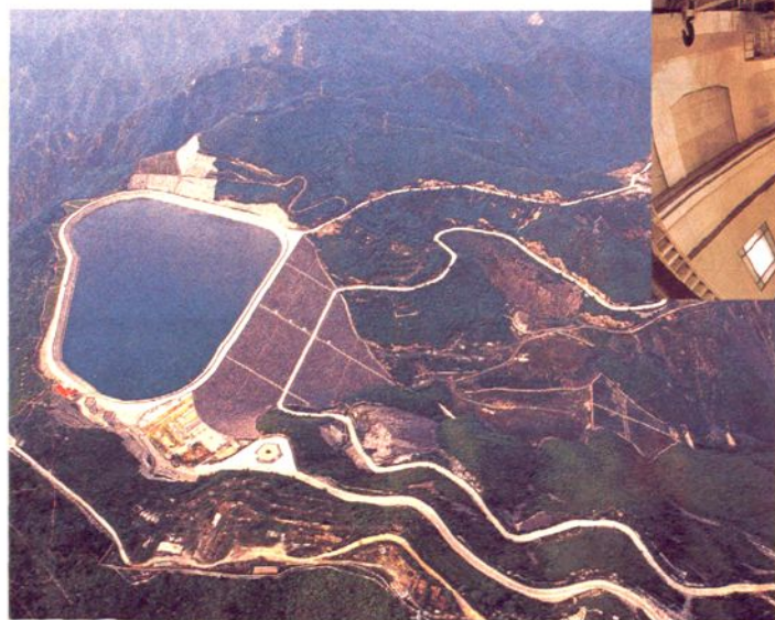
北京十三陵抽水蓄能电站(装机4台，总装机容量80万千瓦)。图为电站上池及地下厂房
