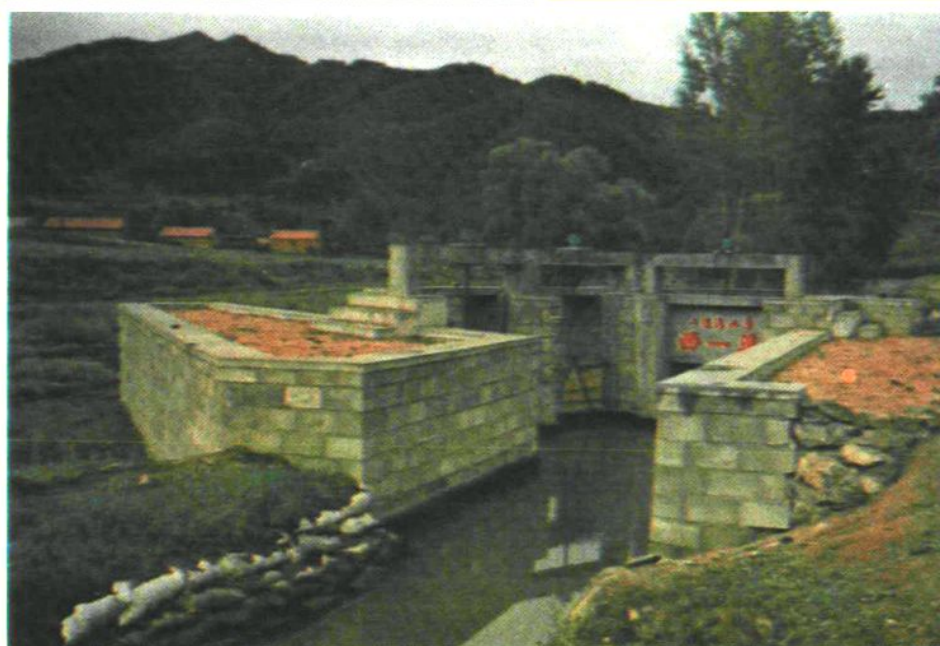
二道湾水库灌渠渠首枢纽工程
