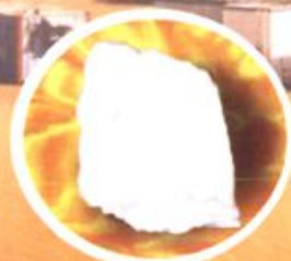
石灰石
