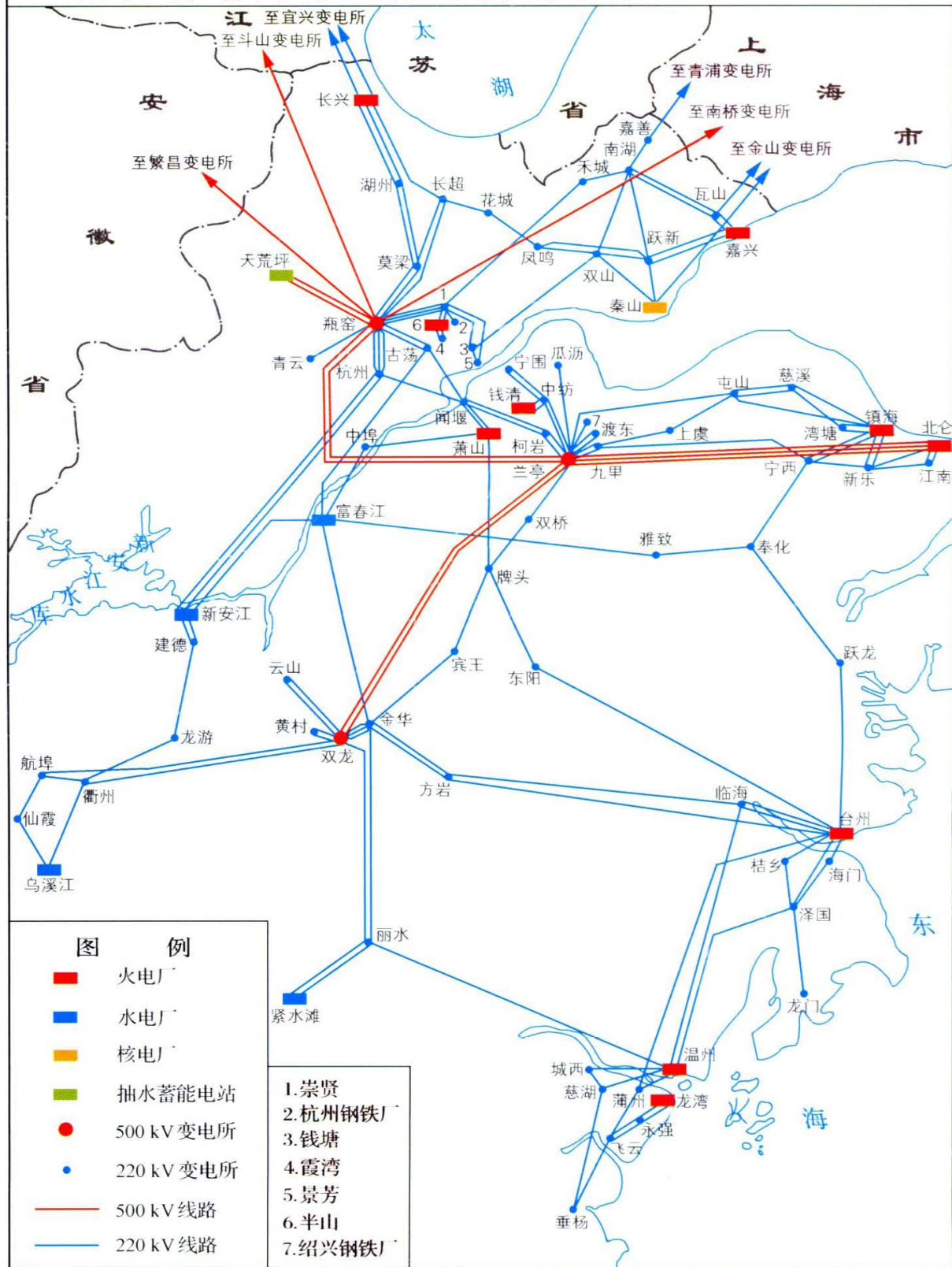
浙江省电网地理位置接线示意图 (1999 年底)
