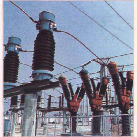
▲ 变电站外景
