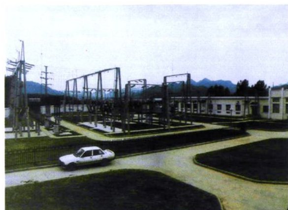
罗庄110千伏变电站
