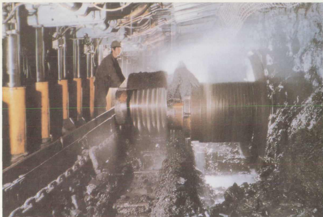
综合机械化采煤
