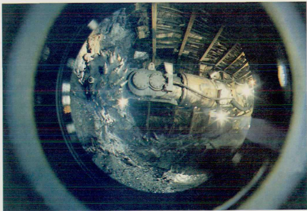
松藻矿务局打通一矿综掘机组
