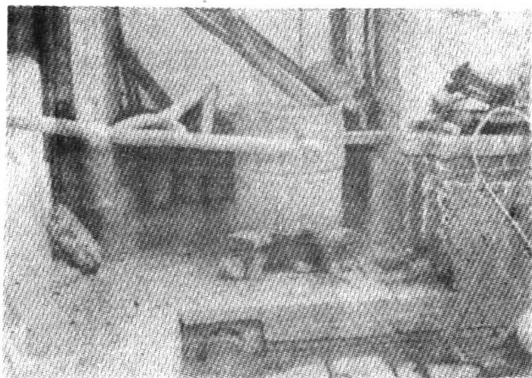
五十年代使用加工大米第一道加工的“累子”
