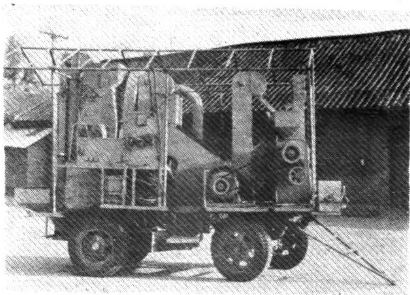
粮油加工厂设计装配的流动式三〇型碾米机
