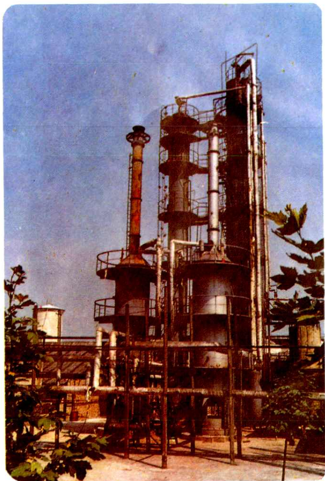
▲ 自贡油毡厂沥青氧化塔
