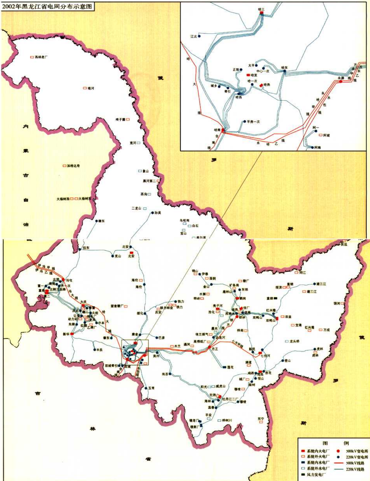
2002年黑龙江省电网分布示意图
