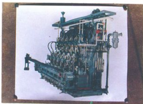
山东省轻工业机械厂生产的Q D 6 行列列制瓶机，自1983年连续 四年被评为轻工业部优质产品。
