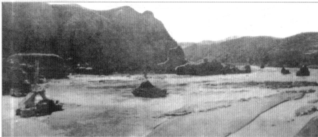
1. 在三门峡坝区峡谷内竖起了一座座钻塔船，日夜不停地在激流中钻探
