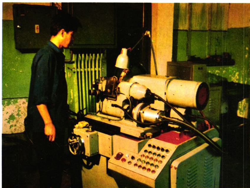
周边磨床
