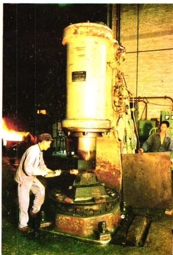
750Kg汽锤
