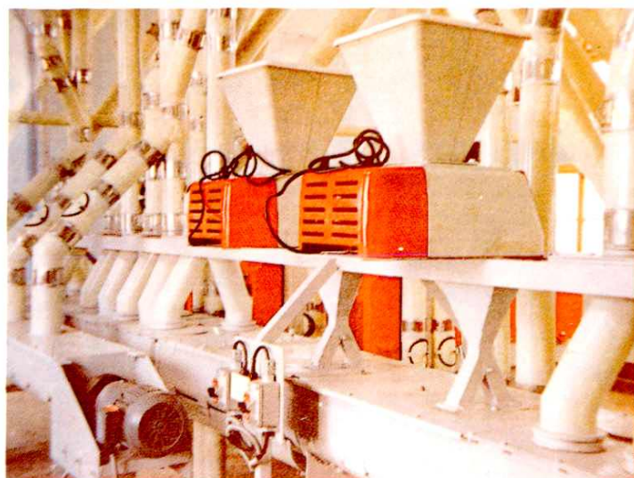
汕头市面粉厂引进意大利面粉生产设备及其产品
