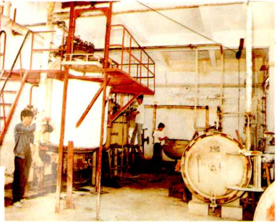
澄海县粮食局蛋白胨厂生产车间
