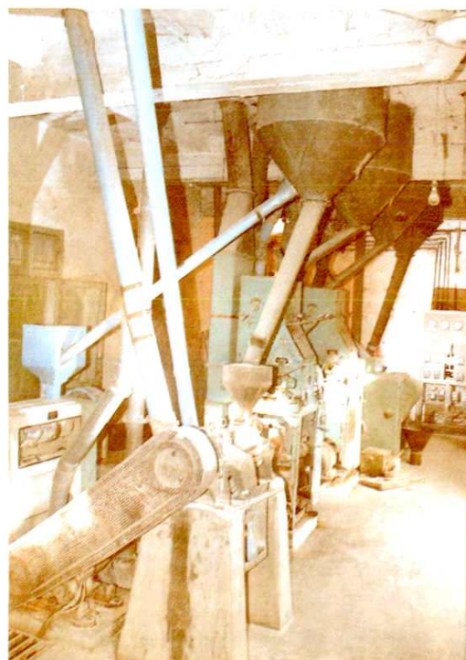
饶平县黄岗粮食加工厂大米车间
