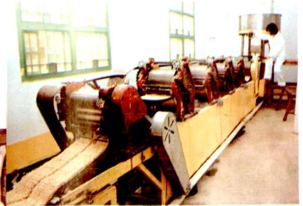
汕头市米面厂波纹面生产线
