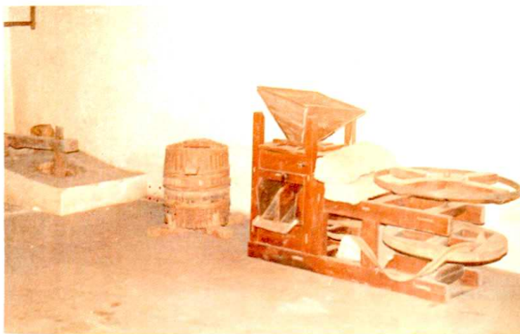
人力加工大米的土碓、土砬、砂砬
