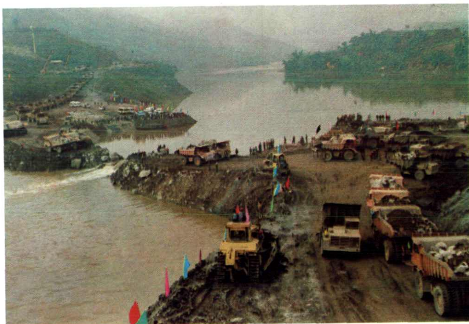
1994年12月25日，天生桥一级电站大坝截流现场
