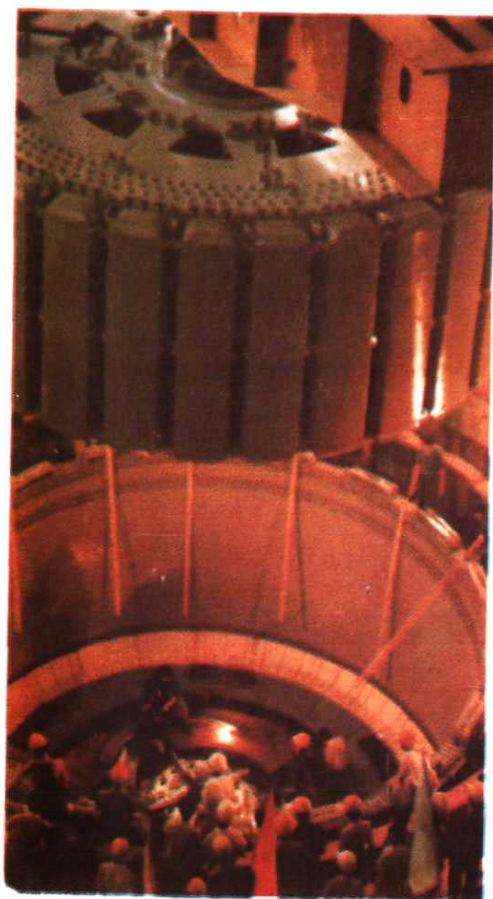
天生桥二级水电站机组转子吊装
