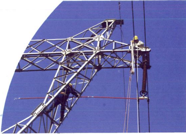
带电更换绝缘子
