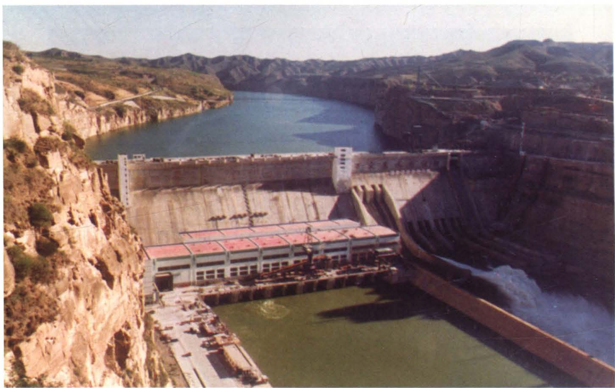
▲ 万家寨引黄入晋工程
