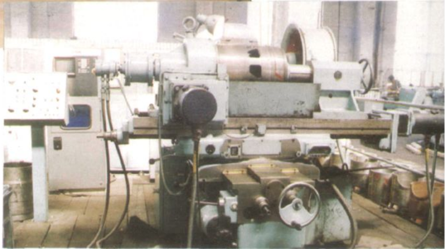
左上 蒸汽机车 整体煮洗工艺 右上 煤水车车 架液压翻转台 左 50吨自动 缩管机
