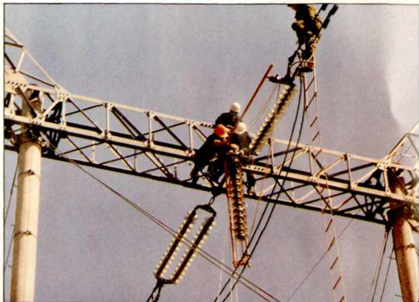
● 带电更换 220 千伏线路耐张绝缘子串
