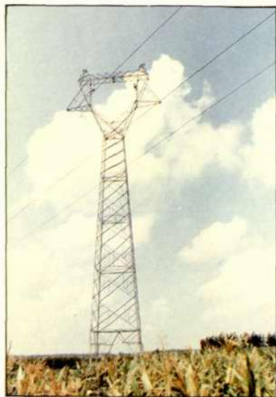
● 架设中的连云港地区第一条 220 千伏 平(墩)——茅(口) 输电线路
