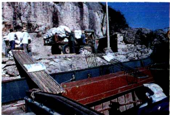
原盐码头装运
