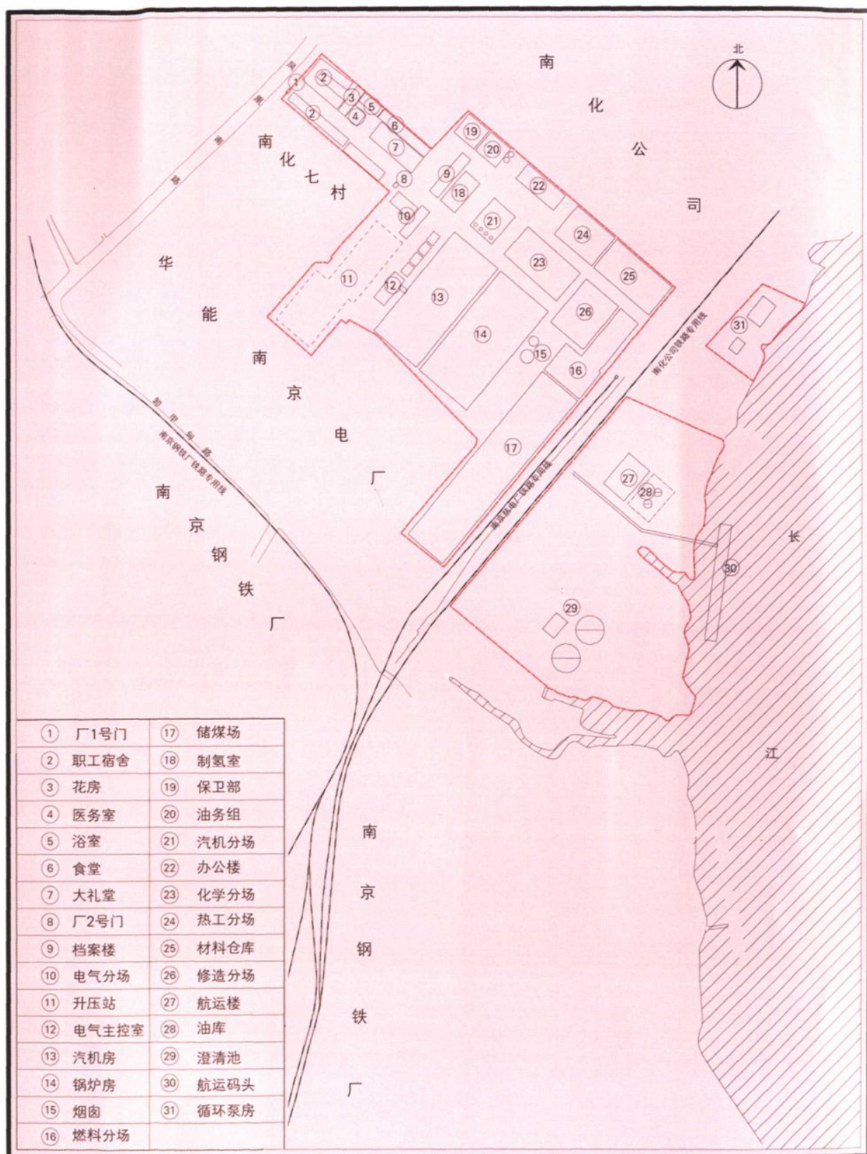
江苏南热发电有限责任公司厂区平面简图 (2005年12月)
