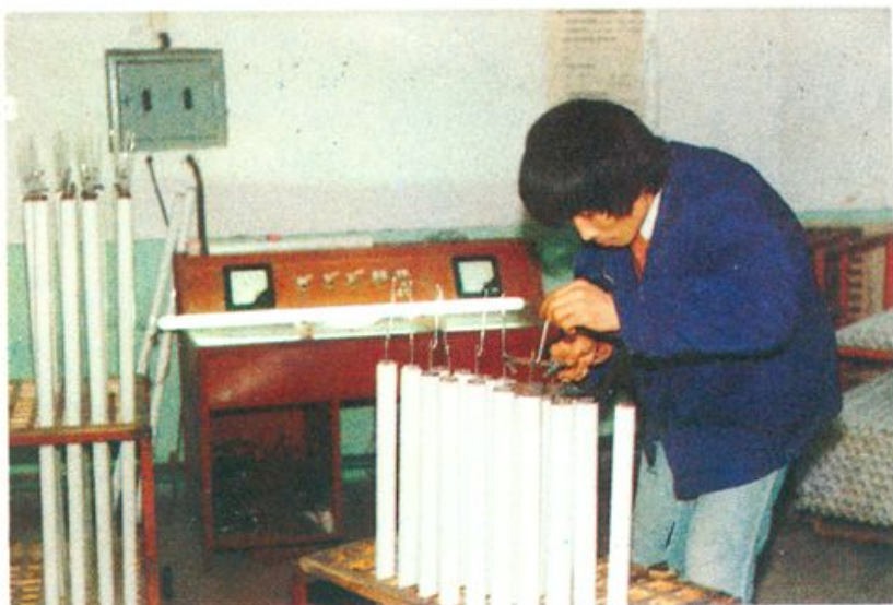
● 水涂粉荧光 灯封口后接排气 管
