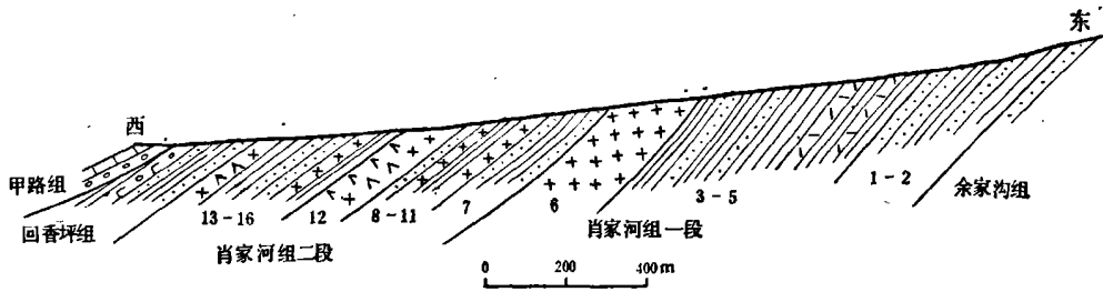
图3 贵州印江肖家河肖家河组剖面略图
