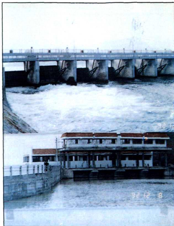
乌溪江引水工程及柯山电站
