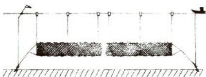
定置刺网作业示意图
