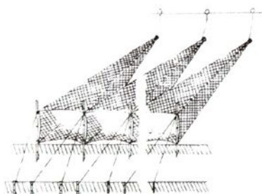
虾户定置张网作业示意图
