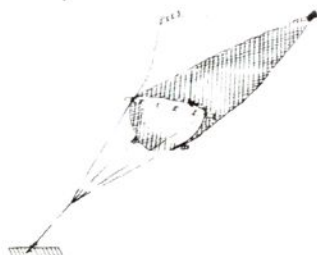
单碇张网作业示意图
