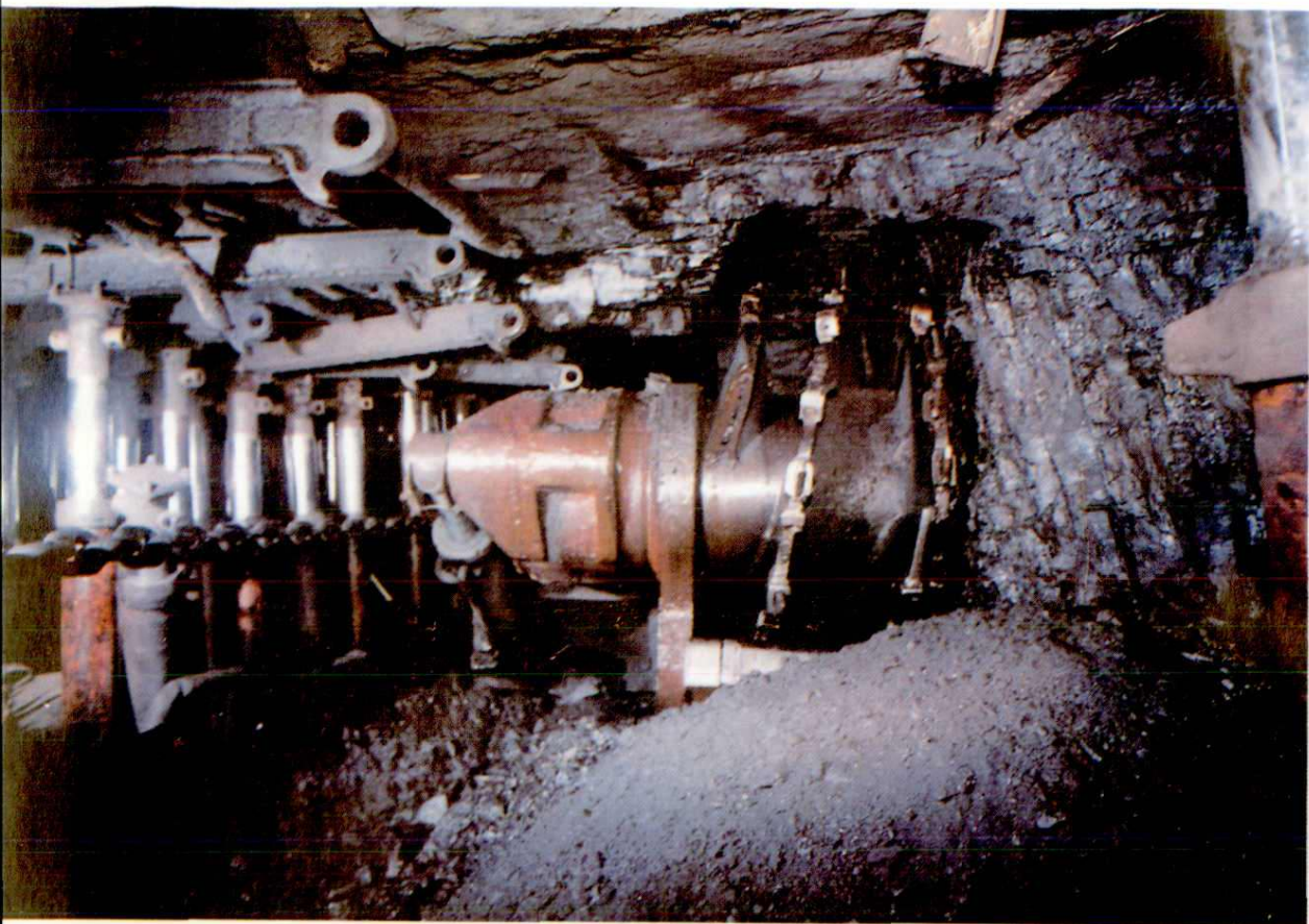
后所煤矿机械化采煤工作面
