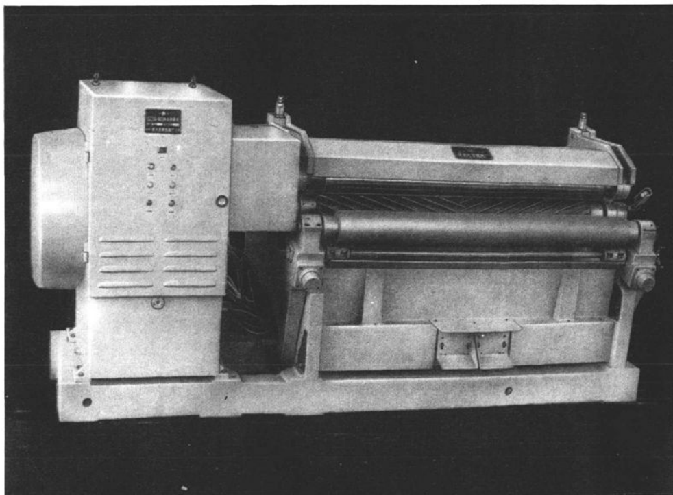
GJ3A1-160挤水伸展机
