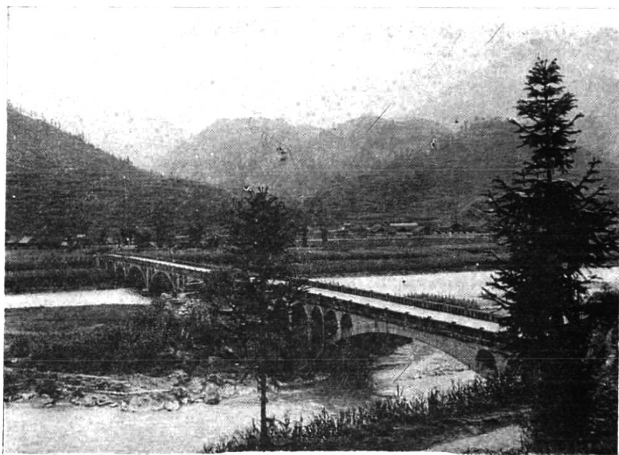
灵关大桥：建于1980年9月，长80米，宽8.5米，横跨于灵关河，连接三个乡（灵关、新兴、大溪）
