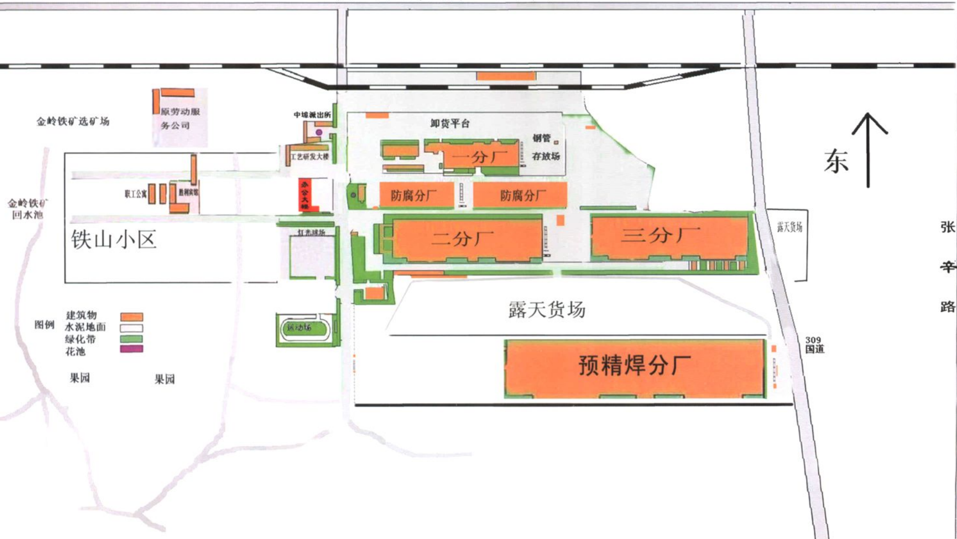
山东胜利钢管有限公司平面示意图
