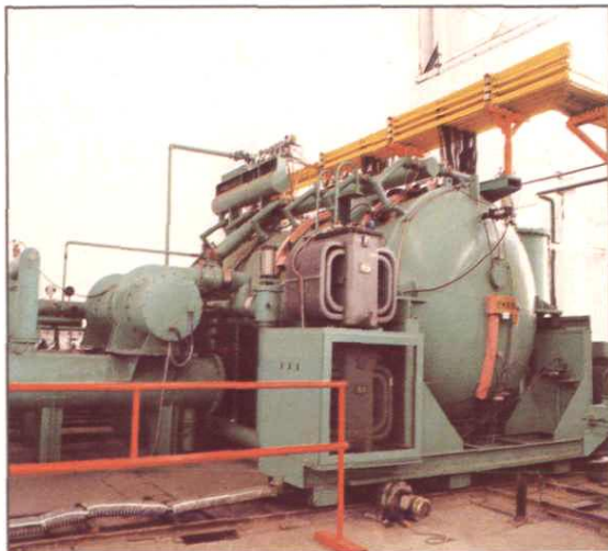
兰州真空设备厂生产的铝板翅式换热器真空钎焊炉(1994年摄)
