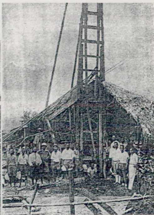
民国20年(1931)8月,高要县石子岗肇南煤矿公司用钻机钻探的情景
