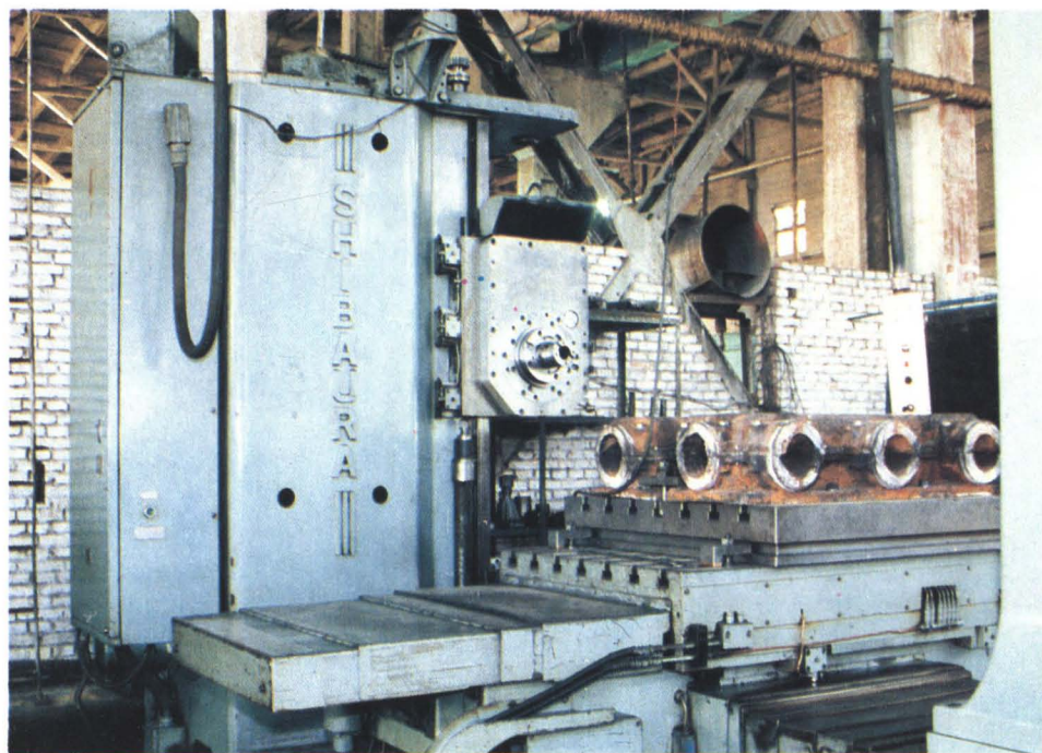
镗床 (T-9)
