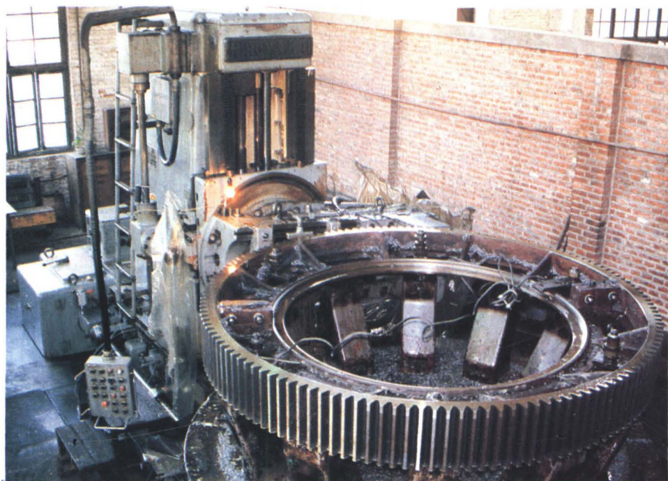
滚齿机 (3.3m)
