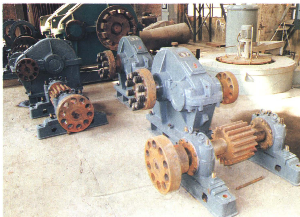
减速器(产品)
