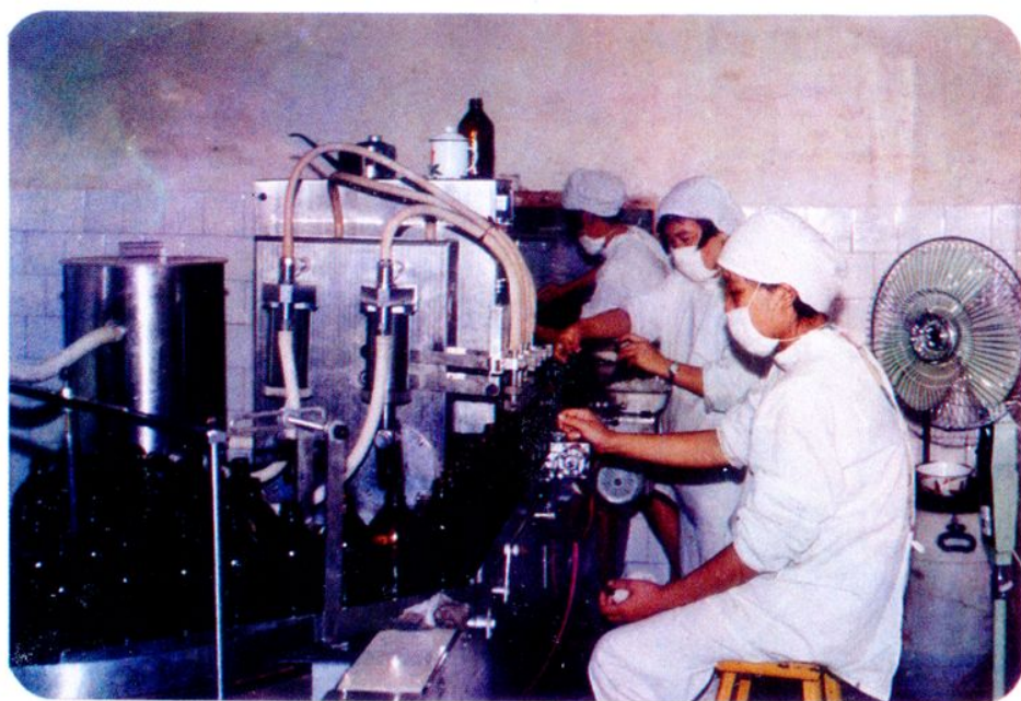
健民制药厂进行技术改造，上图为糖浆灌装线。
