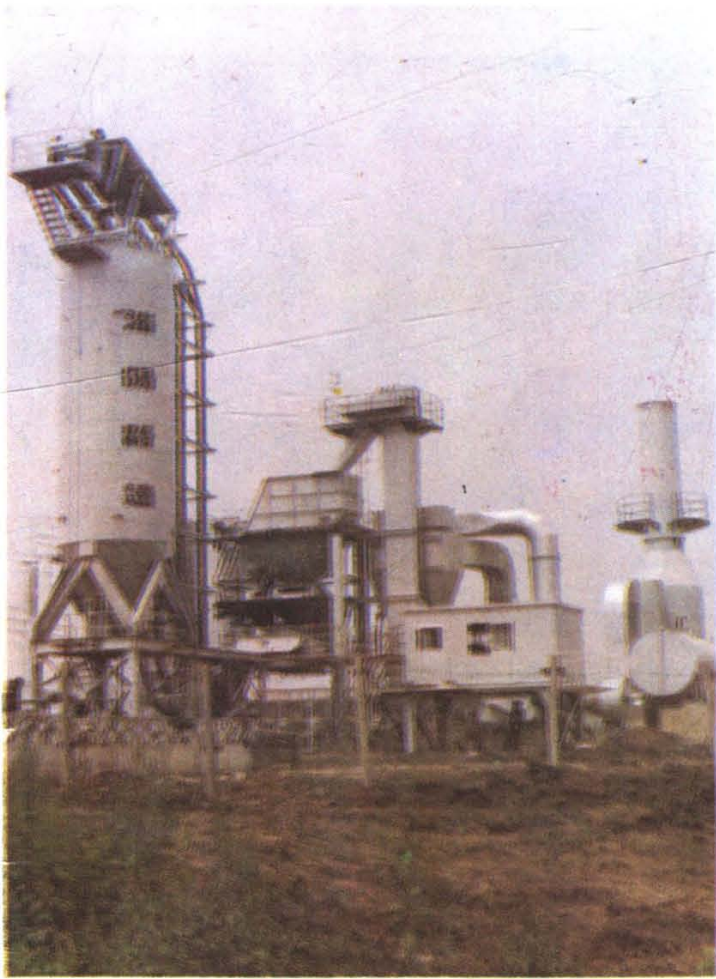
沈阳高等级公路建设总公司下属的沈阳路达筑路机械制造厂研制的 LQB—1200 型沥青混合料拌合设备。
