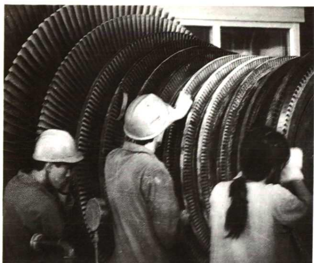
叶片除锈
