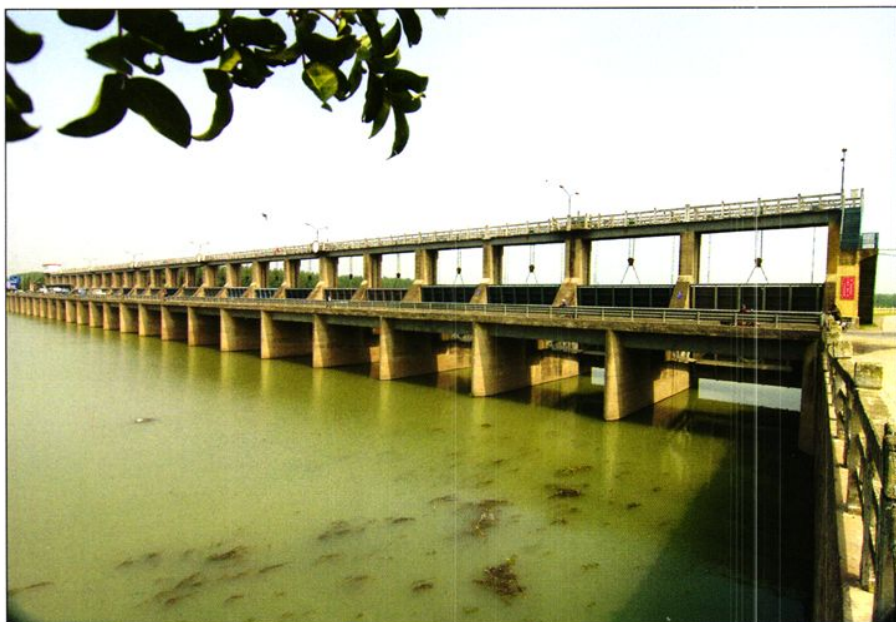
新沂河枢纽沭阳闸工程
