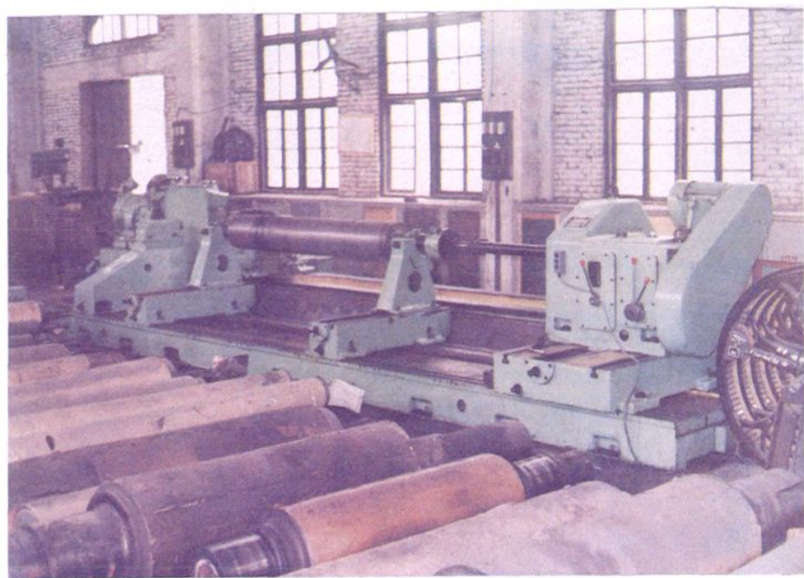
主要设备 之一—— SQZ2805 纸机磨床
