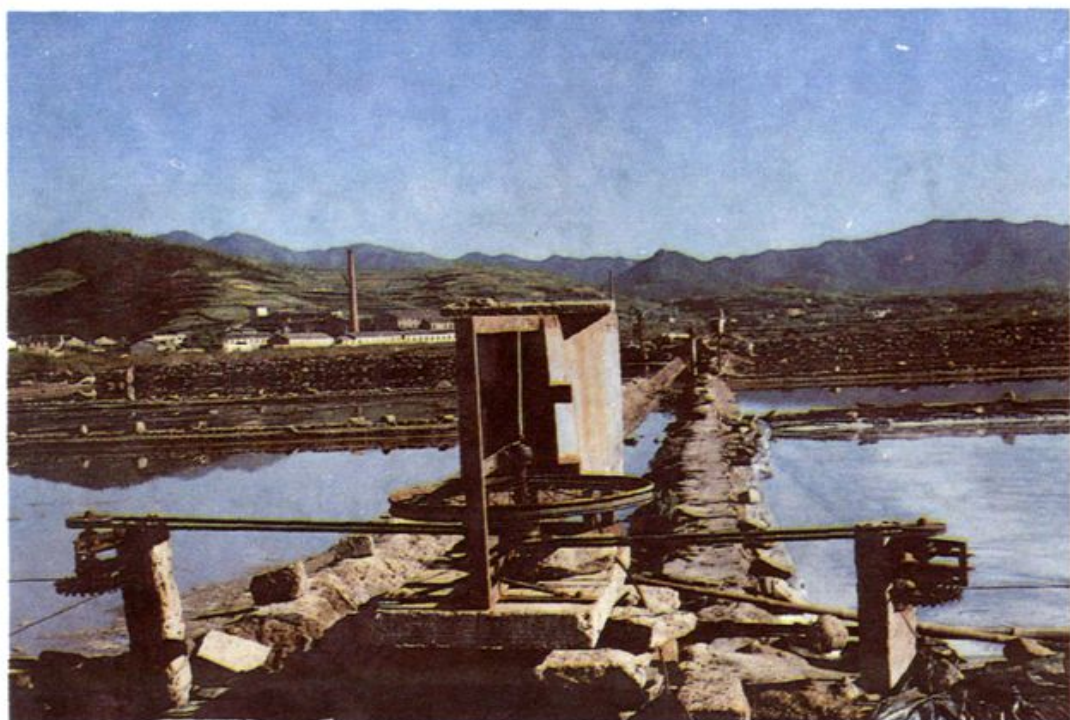
旋卤机
