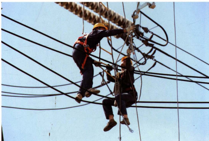
高空作业更换绝缘子串
