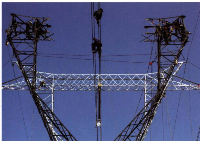
500千伏蔺廉线N145升塔改造
